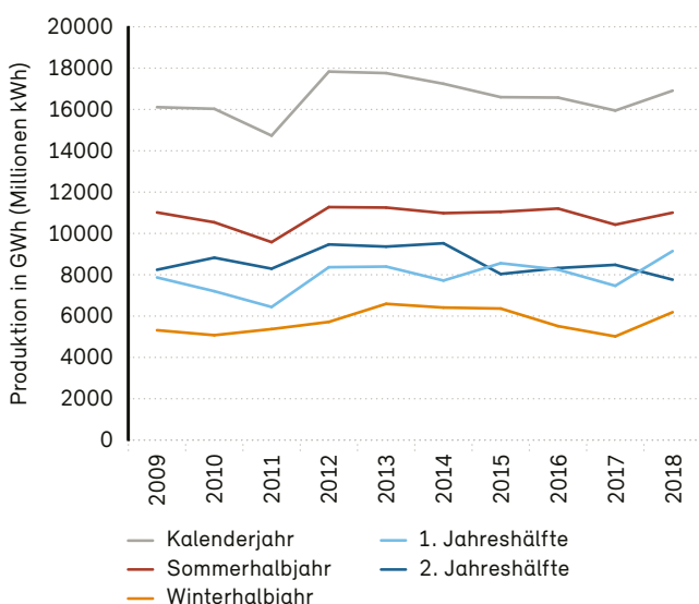
Abb. 29: Stromproduktion der Laufwasserkraftwerke 2009 bis 2018 In der ersten Jahreshälfte 2018 war es das beste Ergebnis und in der zweiten Jahreshälfte das schlechteste Ergebnis der letzten zehn Jahre. Kalenderjahr, Sommerhalbjahr (April bis September), Winterhalbjahr (Oktober bis Dezember des vorhergehenden Jahres sowie Januar bis März des folgenden Jahres)
